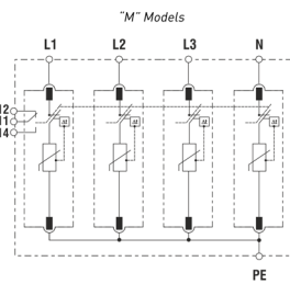
TNS (3Ph+N) - 4P
